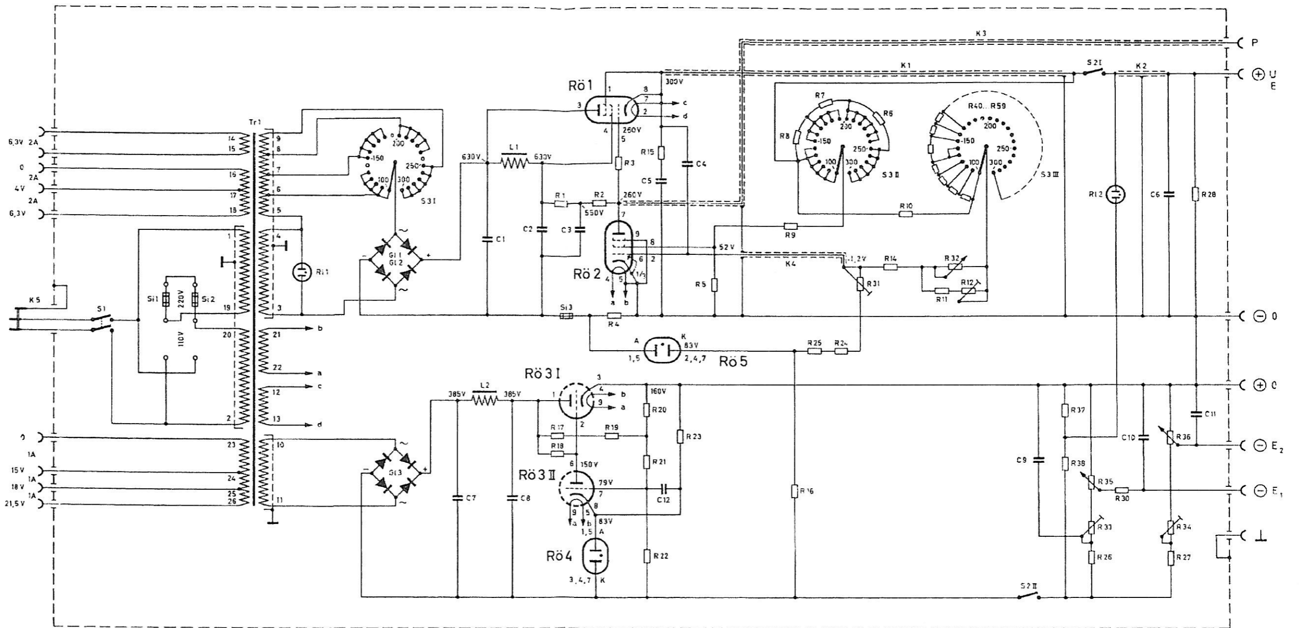
Stromlauf Circuit Diagram
