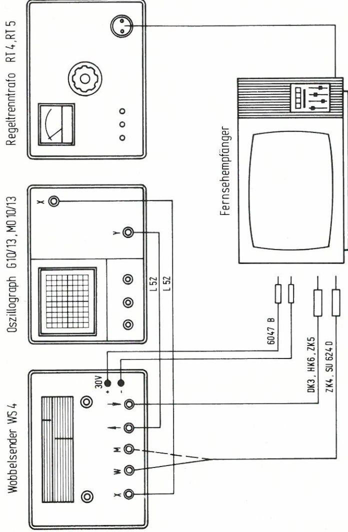
Abb. 2 Anschlußschema
