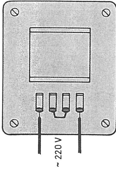
Bild 2: Beschaltung des Netztrafos für 220 V
