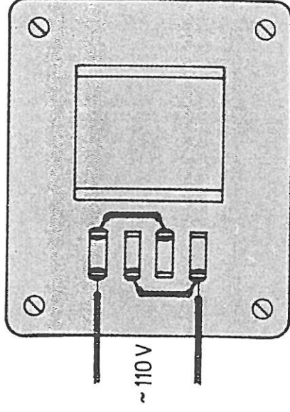
Bild 3: Beschaltung des Netztrafos für 110 V
